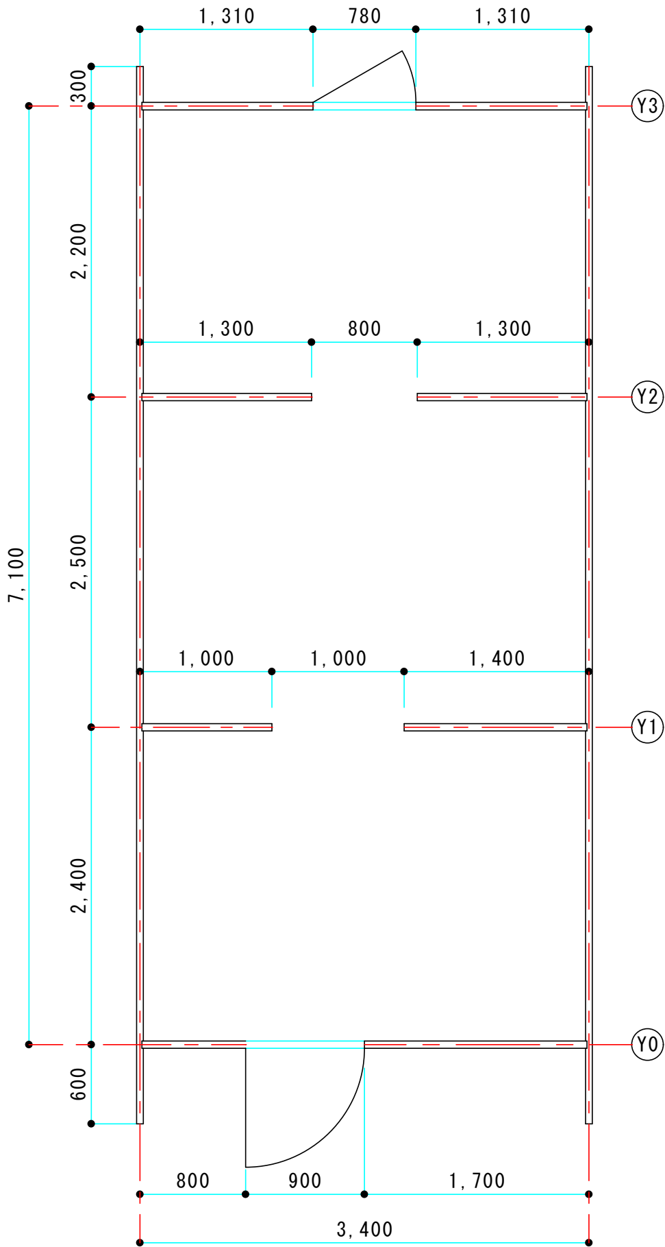
平面图 1/50
